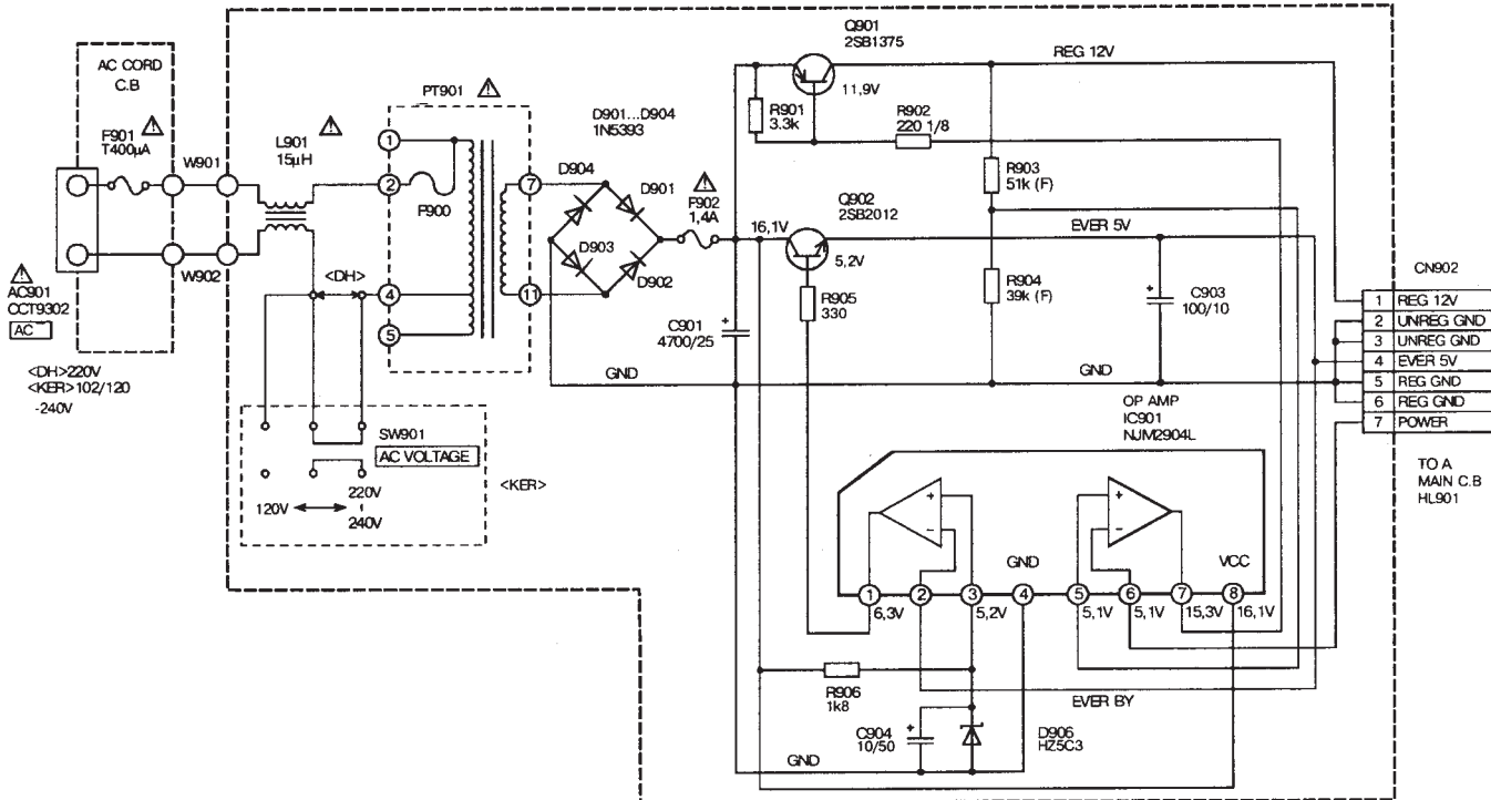
Рис. 2.3. Принципиальная схема источника питания видеоплейеров HV-XE10/XE100.
